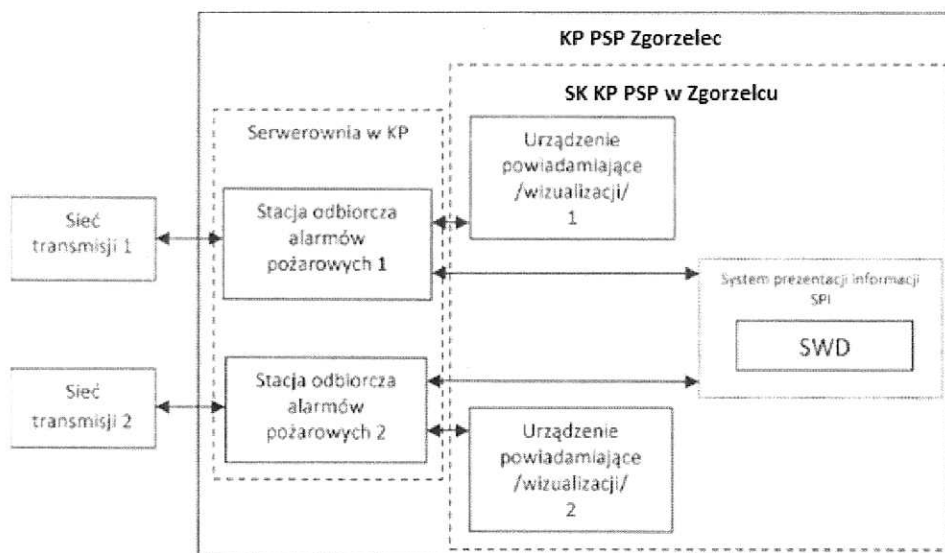
Rys. 3 - Schemat systemu transmisji alarmów pożarowych.
