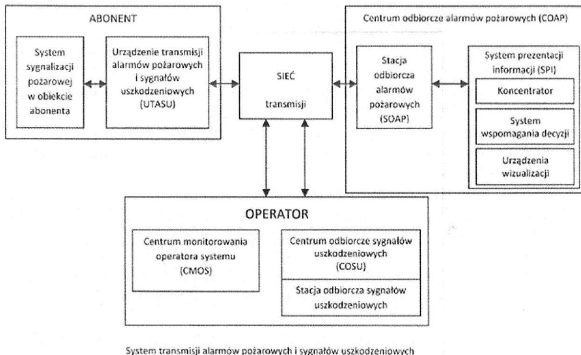
Rys. 1 - Schemat ideowy systemu transmisji alarmów pożarowych i sygnałów uszkodzeniowych — transmisja bezpośrednia
