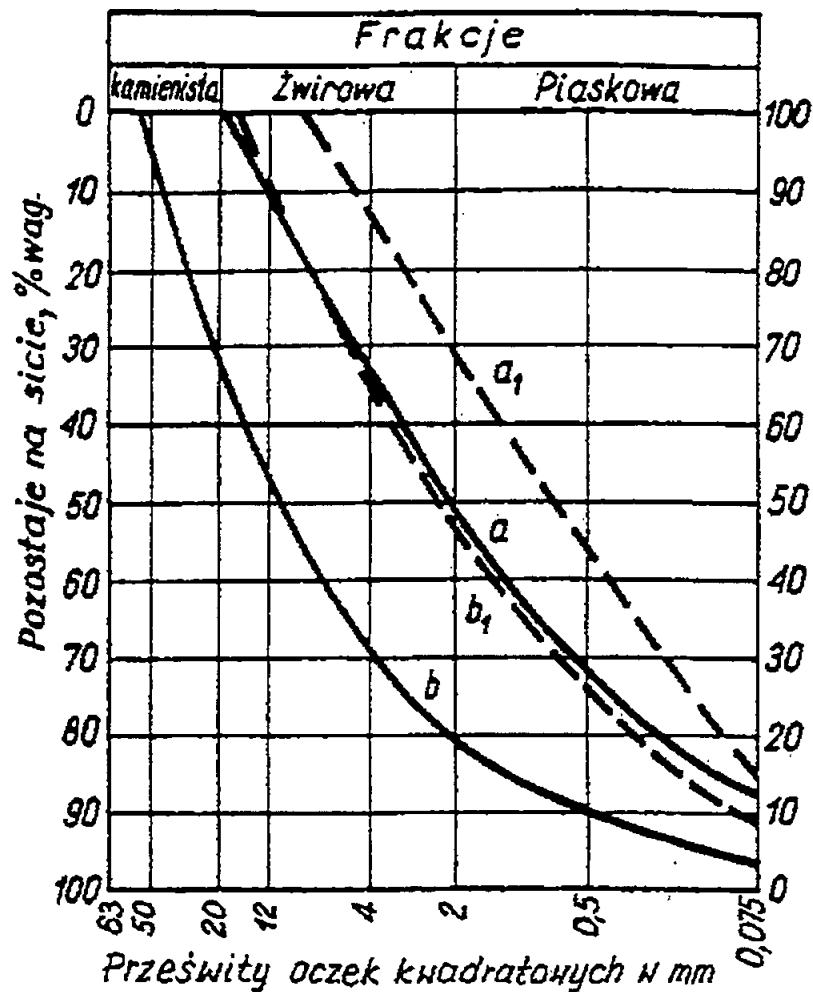
Rysunek 1. Obszar uziarnienia optymalnych mieszanek żwirowych
