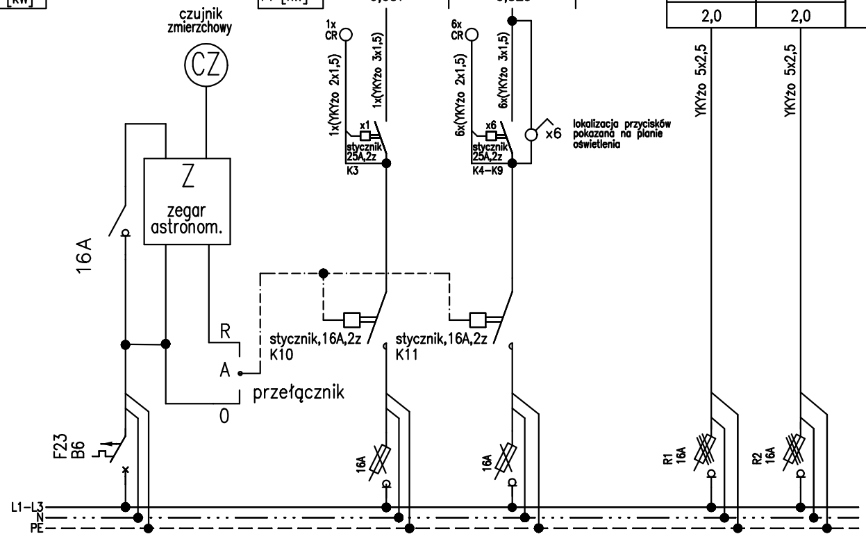
OTE. Część 3 z 3. Układ sieci TN-S
