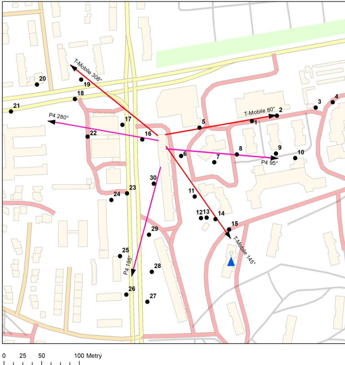
Rys. 1: Plan terenu, na którym znajduje się badane stacje bazowe
