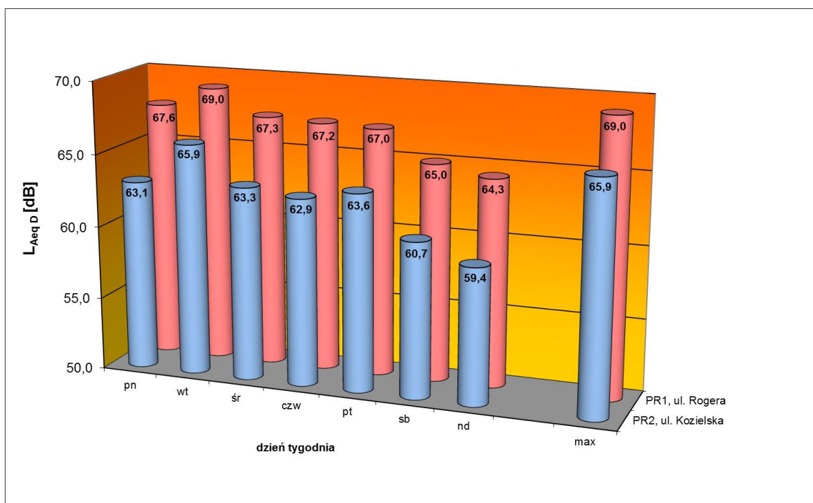
Ryc. 8. Wskaźnik L_{AeqD} (16 h). Zestawienie zmian wskaźnika o wartości maksymalnej poziomu hałasu ( L_{AeqD} ), w danym dniu tygodnia, w ciągu 7-miu dni w badanym roku pomiarów dla przyjętych rejonów badań w Kuźnia Raciborska, 2013 rok, [dB].
