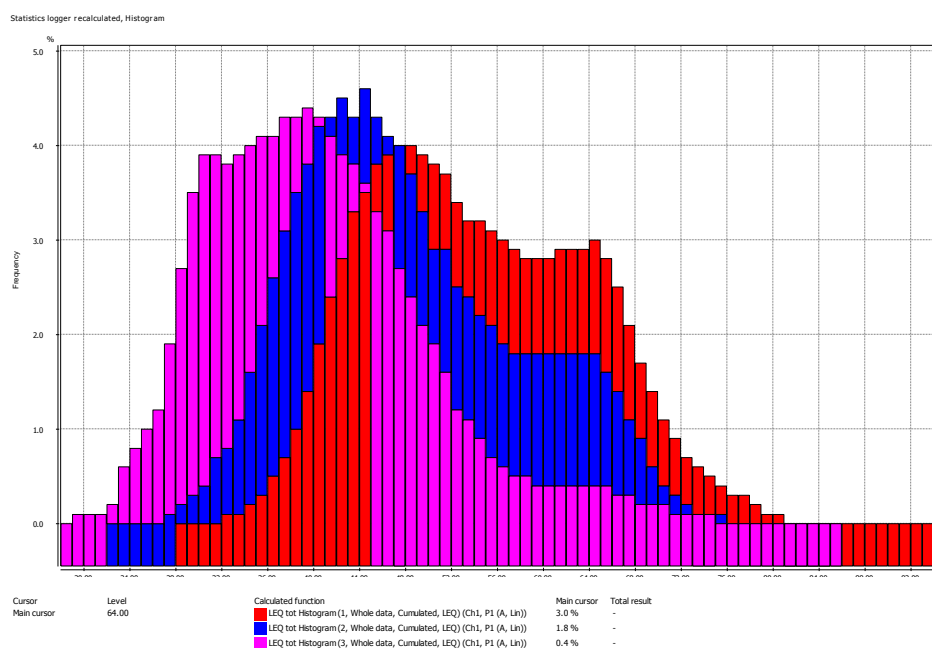
Ryc. 3. Rozkład statystyczny poziomów dźwięku hałasu drogowego dla pory dnia (kol. czerwony), pory wieczoru (kol. zielony) i pory nocy (kol. granatowy) w pkt. pom. PR2 - ul. Kozielska, Kuźnia Raciborska, 2013 r. (z sesji tygodniowej).
