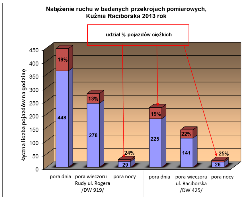
Ryc. 12. Procentowy udział pojazdów ciężkich w potoku ruchu w badanych punktach, Kuźnia Raciborska 2013 rok.
