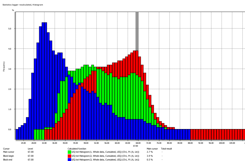
Ryc. 2. Rozkład statystyczny poziomów dźwięku hałasu drogowego dla pory dnia (kol. czerwony), pory wieczoru (kol. zielony) i pory nocy (granatowy) w pkt. pom. PR1 – ul. Rogera, Rudy, 2013 r. (z sesji tygodniowej).
