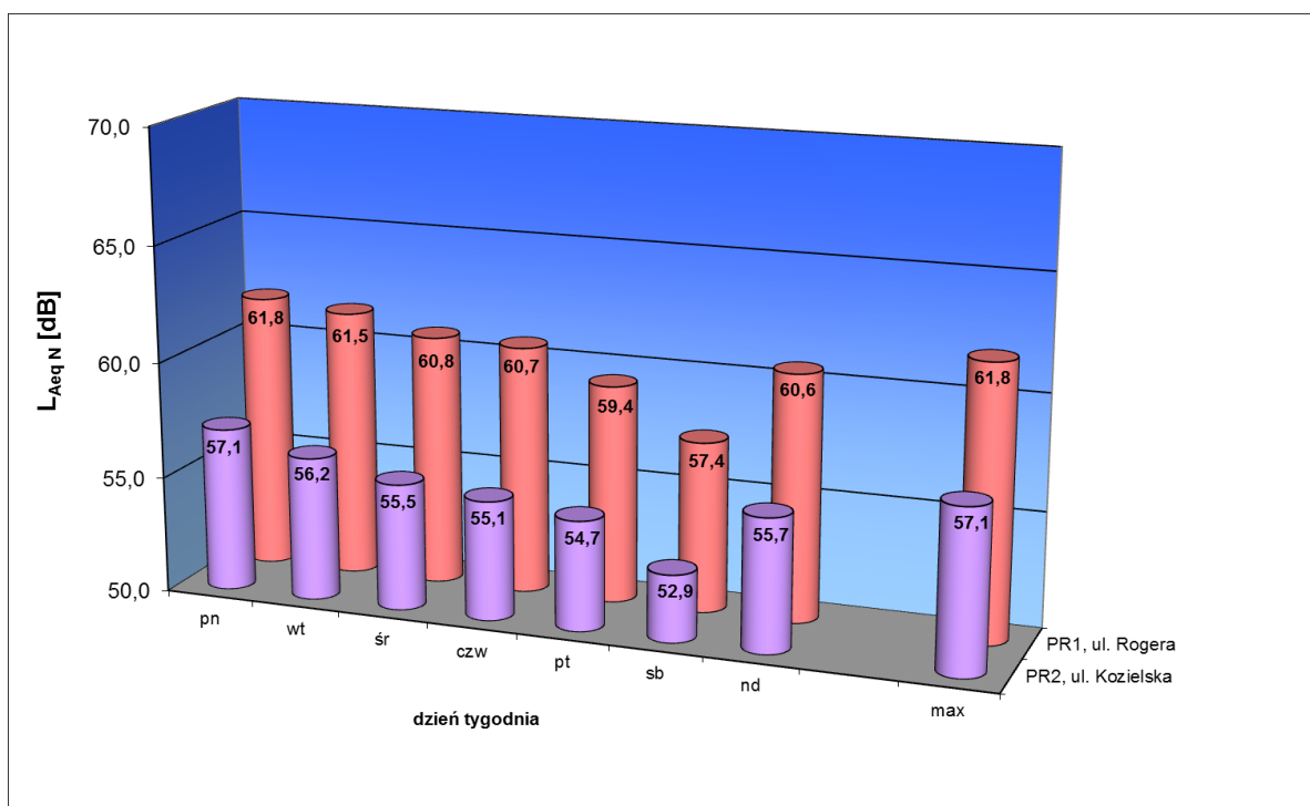
Ryc. 9. Wskaźnik L_{AeqN} (8 h). Zestawienie zmian wskaźnika o wartości maksymalnej poziomu hałasu ( L_{AeqN} ), w danym dniu tygodnia, w ciągu 7-miu dni w badanym roku pomiarów dla przyjętych rejonów badań w Kuźnia Raciborska, 2013 rok, [dB].
