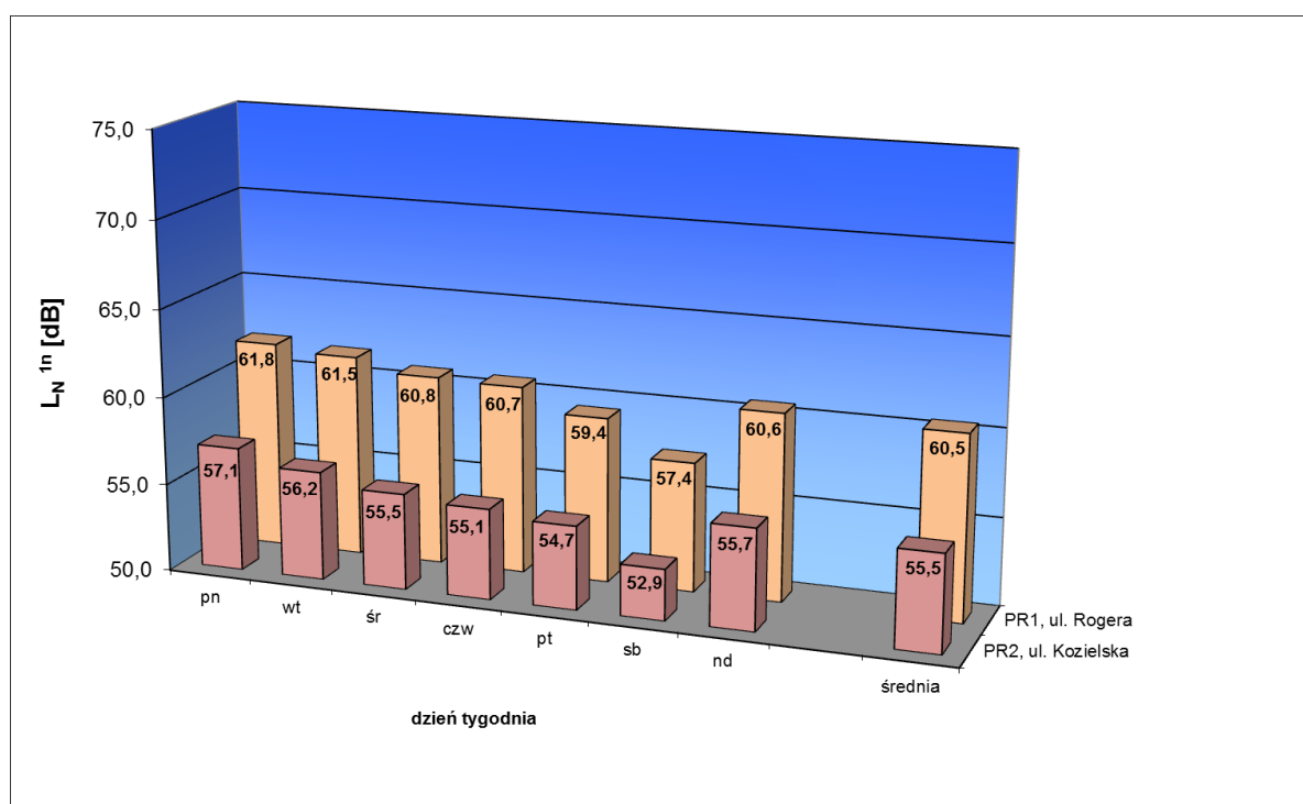
Ryc. 5. Wskaźnik L_N^{1n} (8 h) w [dB]. Zestawienie zmian wskaźnika dla pory nocy ( L_N ) z poszczególnych nocy z 1 tygodniowej sesji pomiarowej wraz z wartością średnią tygodniową, Kuźnia Raciborska, 2013 r.
