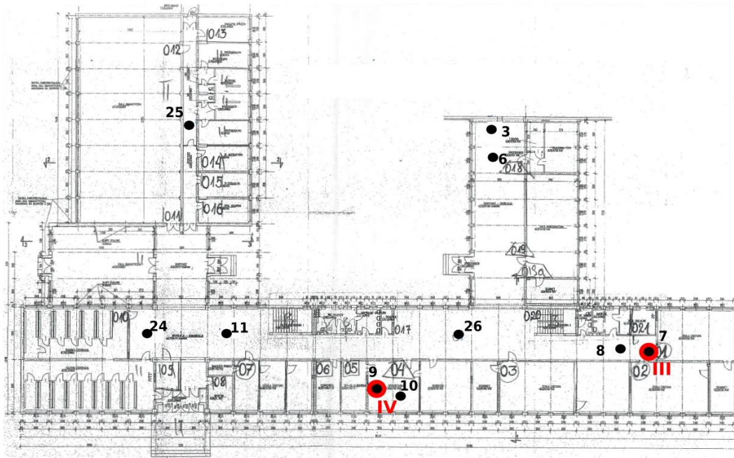
Rys. 1b: Plan rozmieszczenia punktów pomiarowych – parter, kolorem czerwonym oznaczono lokalizację punktów dostępnych
