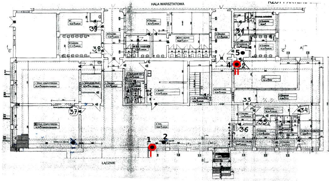
Rys. 1a: Plan rozmieszczenia punktów pomiarowych – parter, część administracyjna kolorem czerwonym oznaczono lokalizację punktów dostępnych
