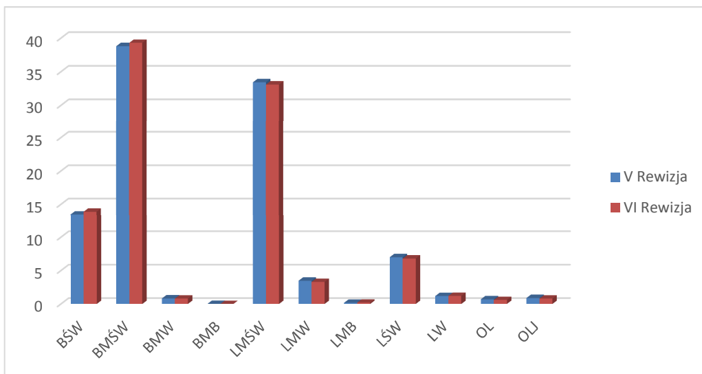
Wykres 3. Procentowe zmiany powierzchni typów siedliskowych lasu IV i V rewizji PUL
