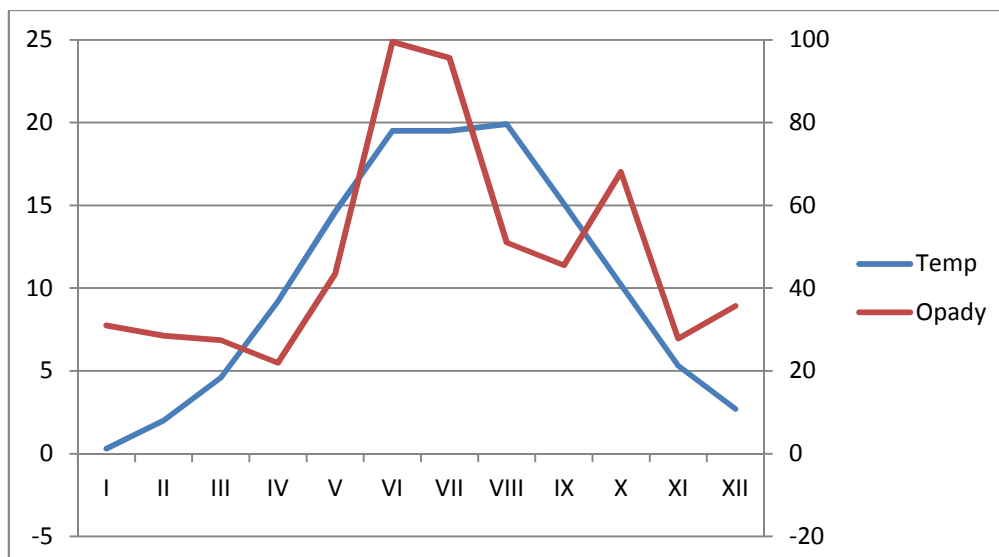
Wykres 1. Opady i temperatura
