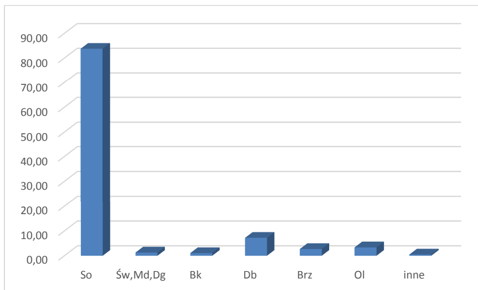
Wykres 8 Udział miąższociowy panujących gatunków drzew w procentach
