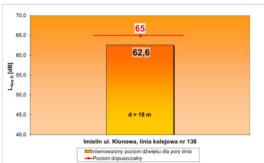
Ryc. 2. Wartość wskaźnika L_{Aeq D} dla rozpatrywanego punktu referencyjnego oraz jego porównanie z obowiązującą wartością poziomu dopuszczalnego, Imielin, 2022 rok.
