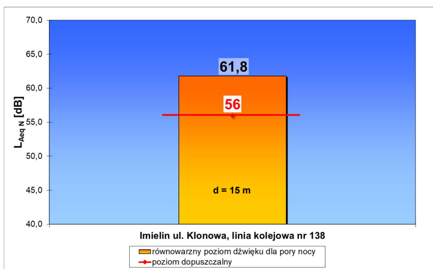
Ryc. 3. Wartość wskaźnika L_{Aeq N} dla rozpatrywanego punktu referencyjnego oraz jego porównanie z obowiązującą wartością poziomu dopuszczalnego, Imielin, 2022 rok.
