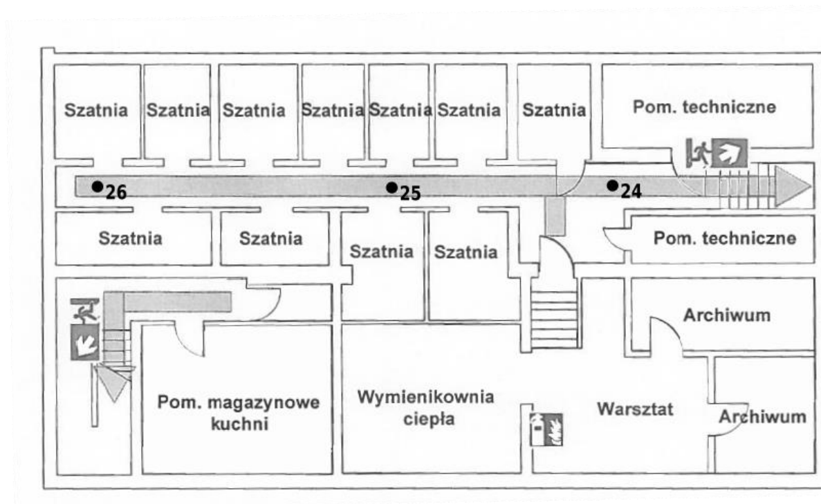
Rys. 1d: Plan rozmieszczenia punktów pomiarowych – piwnica
