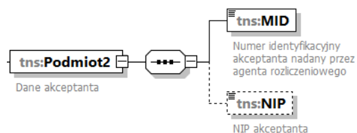
Schemat 7. Struktura Podmiot2 w ITP-Z.
