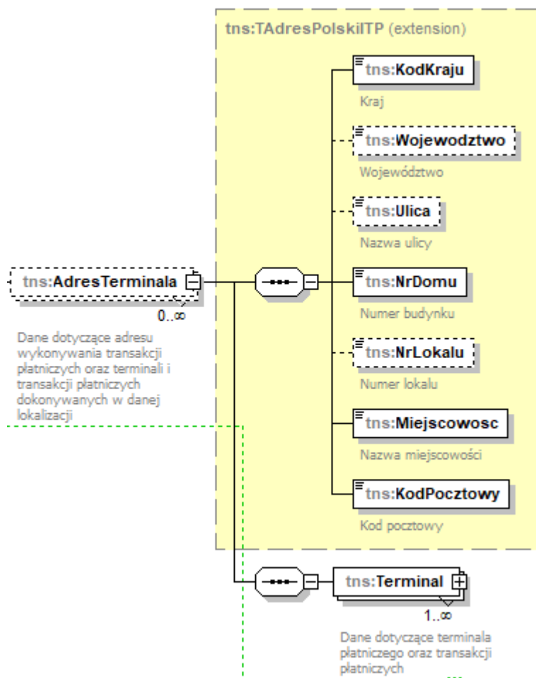
Schemat 9. Struktura adresu terminala w ITP-Z.
