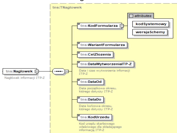
Schemat 2. Struktura nagłówka w ITP-Z.
