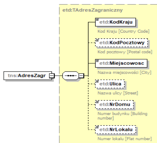
Schemat 6. Struktura adresu zagranicznego agenta rozliczeniowego w ITP-Z.
