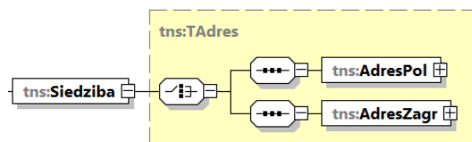
Schemat 4. Struktura adresu siedziby agenta rozliczeniowego w ITP-Z.
