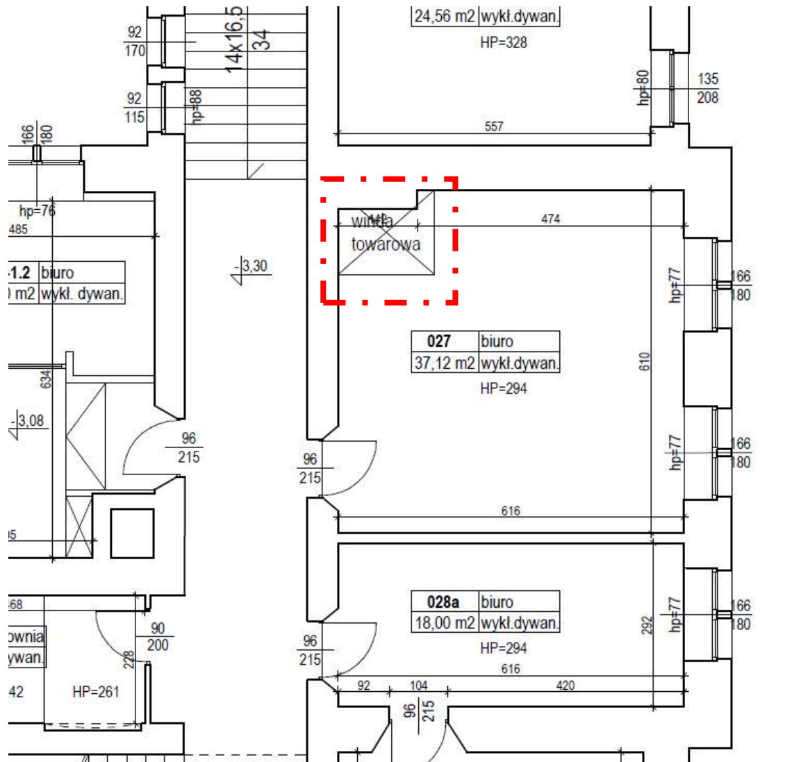
Rys. Nr 2 Fragment rzutu przyziemia – pokój nr 027.
