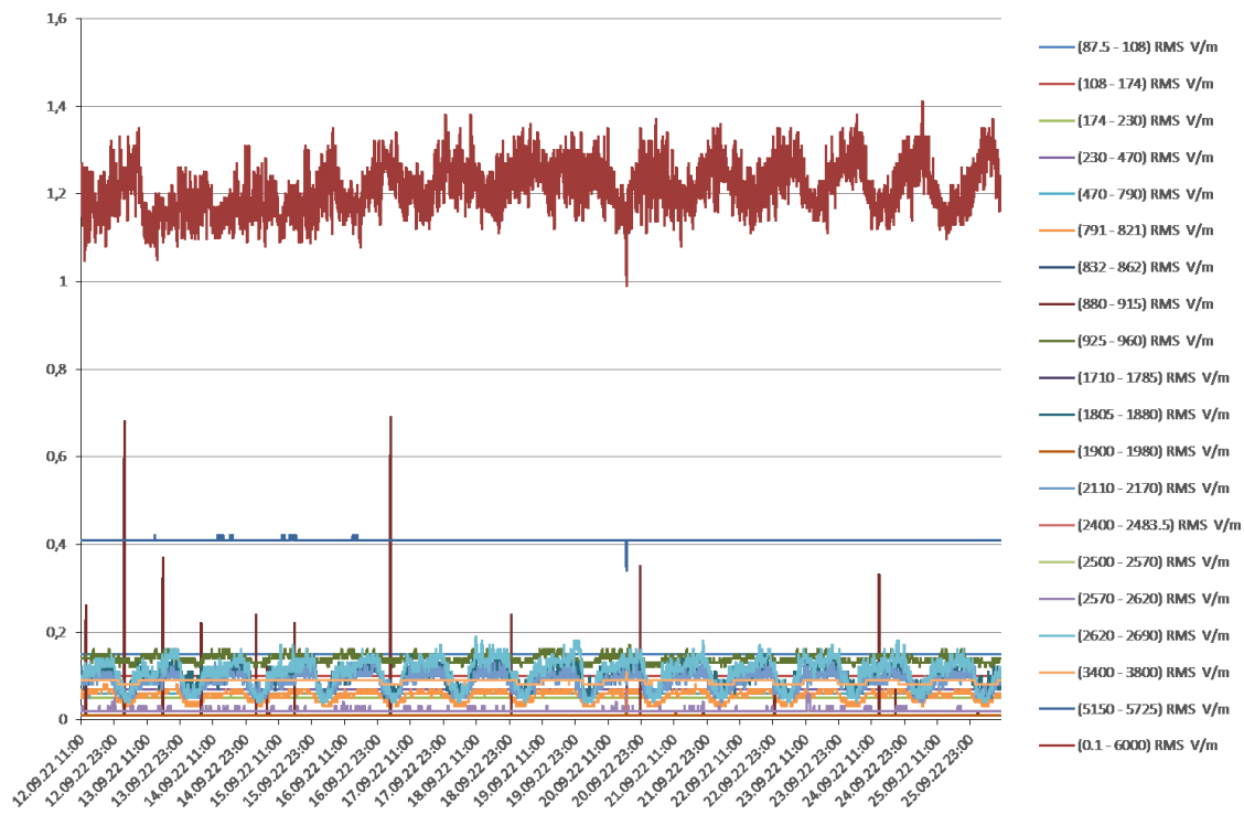
Rys. 5 Wyniki pomiarów dla 20 podzakresów częstotliwości – Szkoła Podstawowa nr 10 w Pruszkowie
