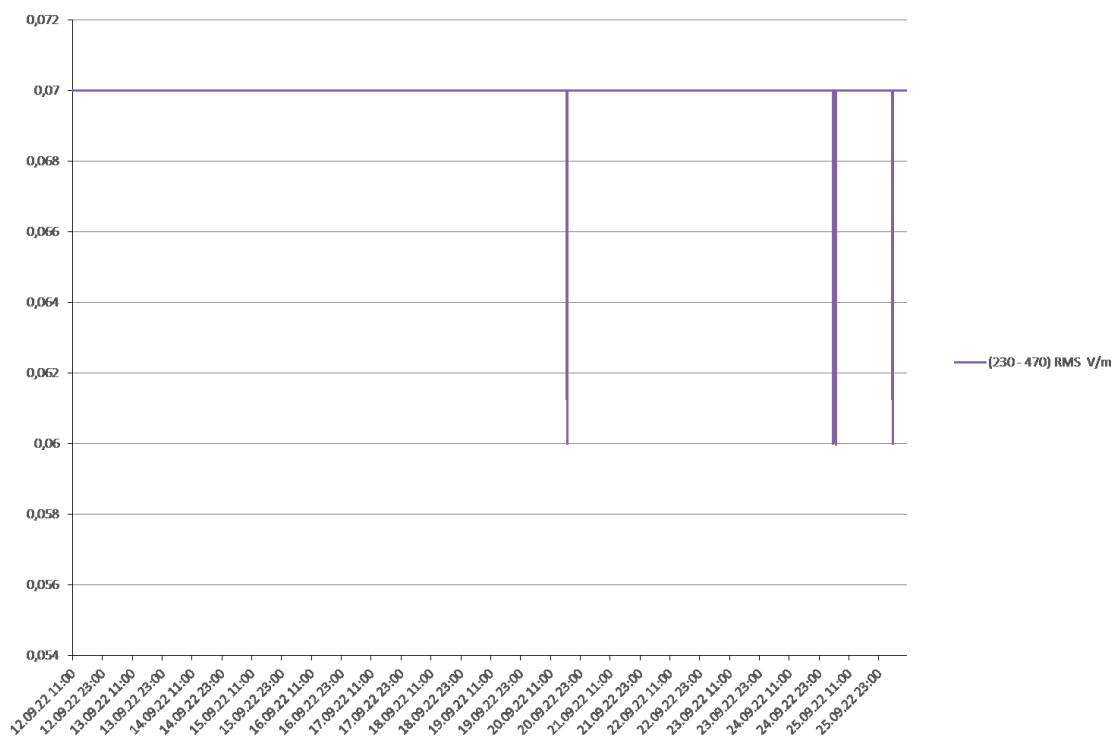
Rys. 10 Wyniki pomiarów w zakresie częstotliwości: 230,0 MHz – 470,0 MHz
