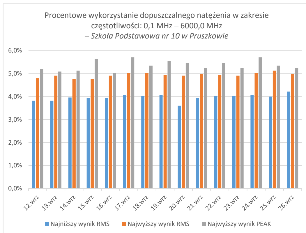
Rys. 26 Procentowe wykorzystanie dopuszczalnego natężenia w zakresie częstotliwości: 0,1 MHz – 6000,0 MHz – Szkoła Podstawowa nr 10 w Pruszkowie
