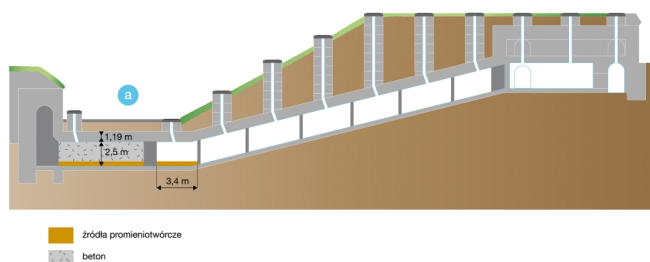
Rys. 2. Obiekt 3a przeznaczony do składowania zużytych zamkniętych źródeł promieniotwórczych [1].
