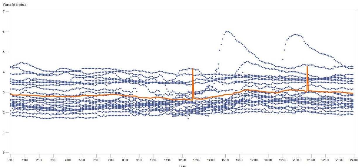
Rys. 8 Wyniki pomiarów – UM Łódź– średnia za okres 24 godzin
