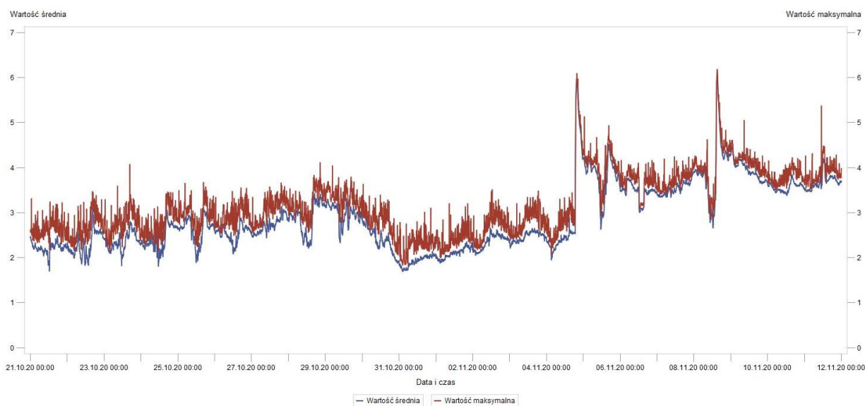
Rys. 6 Wyniki pomiarów – UM Łódź w okresie 21.10.2020 r. – 11.11.2020 r.
