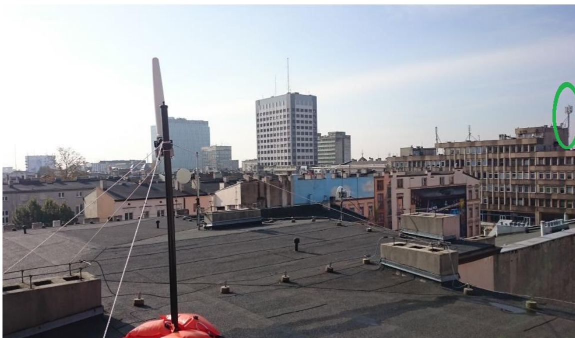
Rys. 2 Miejsce montażu pilotażowego SMS PEM – dach UM Łódź – widok na anteny SBTK
