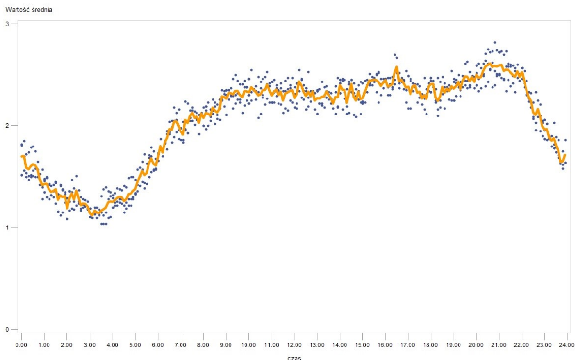
Rys. 6 Wyniki pomiarów – MOSiR „Bystrzyca” w Lublinie – średnia za okres 24 godzin
