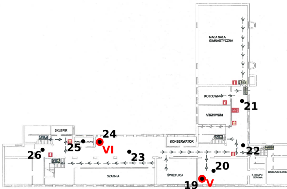
Rys. 1c: Plan rozmieszczenia punktów pomiarowych – piwnica, kolorem czerwonym oznaczono lokalizacje punktów dostępowych
