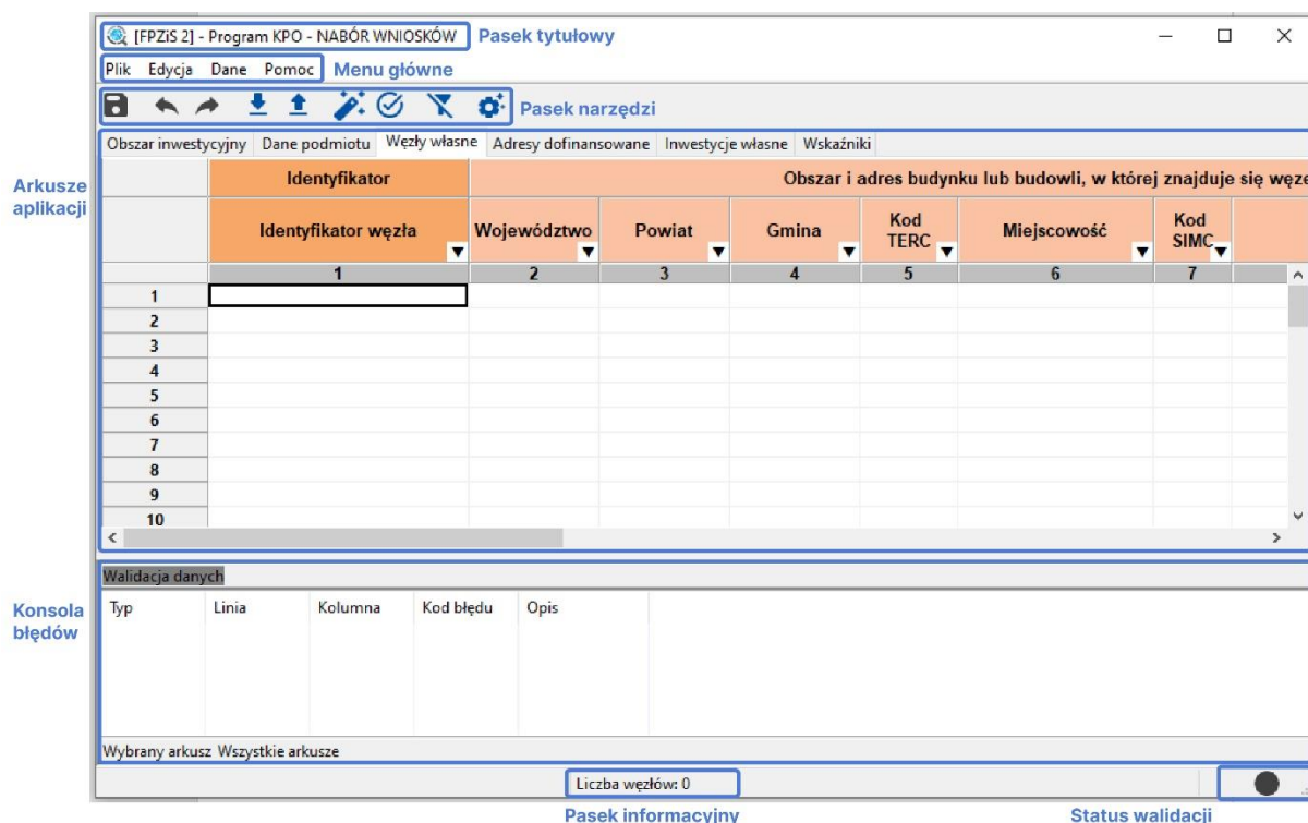
Rys. 1. Aplikacja FPZIS 2
