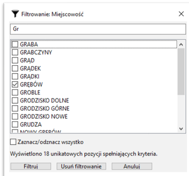
Rys. 18. Przykładowe filtrowanie
