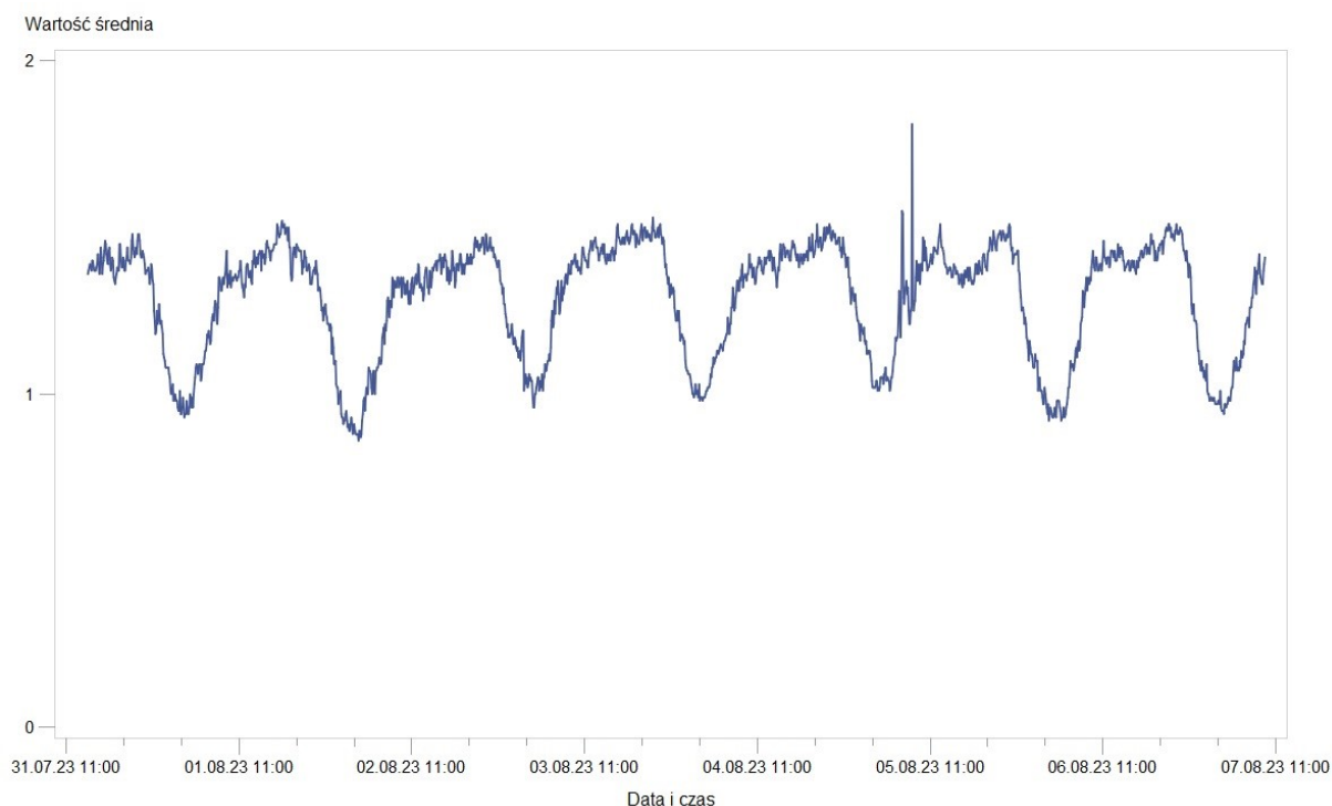
Rys. 5 Wyniki pomiarów – Szkoła Podstawowa nr 6 w Mielcu w dniach 31.07.2023 r. – 7.08.2023 r. – wartość średnia
