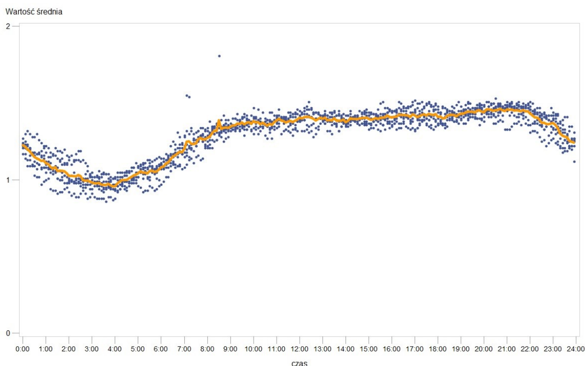
Rys. 7 Wyniki pomiarów – Szkoła Podstawowa nr 6 w Mielcu – średnia za okres 24 godzin
