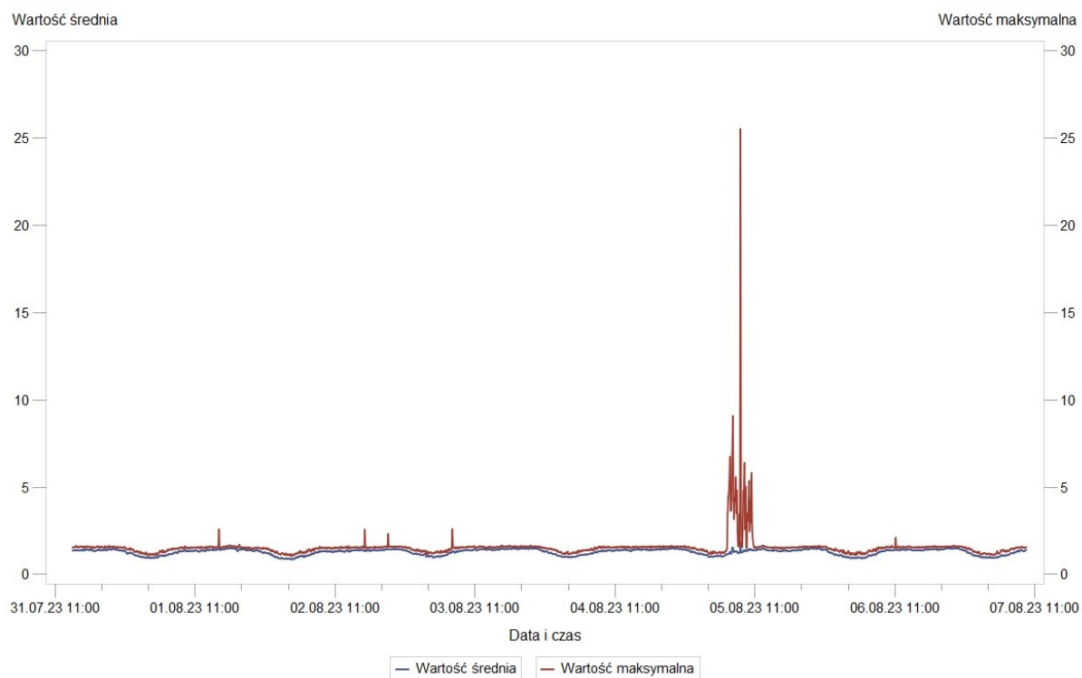
Rys. 6 Wyniki pomiarów – Szkoła Podstawowa nr 6 w Mielcu w dniach 31.07.2023 r. – 7.08.2023 r. – wartość średnia i wartość maksymalna
