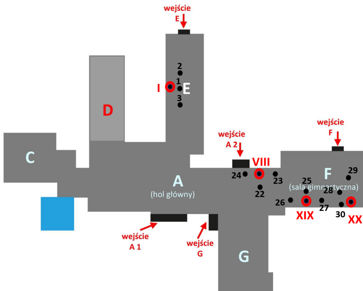
Rys. 1b: Plan rozmieszczenia punktów pomiarowych – Parter, kolorem czerwonym oznaczono lokalizację punktów dostępnych
