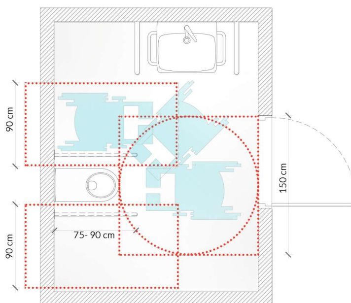
Rys. 54 Toaleta przeznaczona dla osób z niepełnosprawnościami
