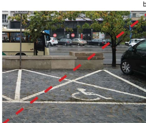
Zdj. 01 Nawierzchnia miejsca postojowego dla osób z niepełnosprawnością zdj. a: równa i gładka kostka betonowa – zalecana, zdj. b: bruk kamienny - rozwiązanie niepoprawne
