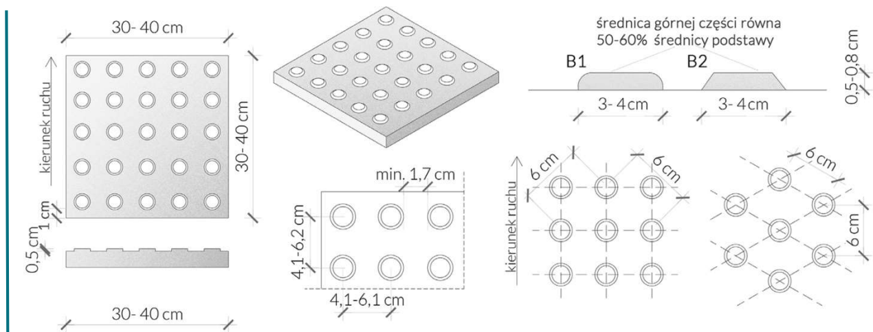
Rys. 23 Faktura bezpieczeństwa (typ B) tzw. B1 „ścięte kopułki”, B2 „ścięte stożki”.
