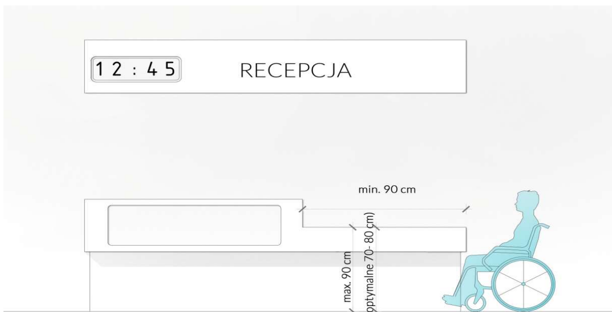
Rys. 44 Wytyczne dotyczące dostępności lad
