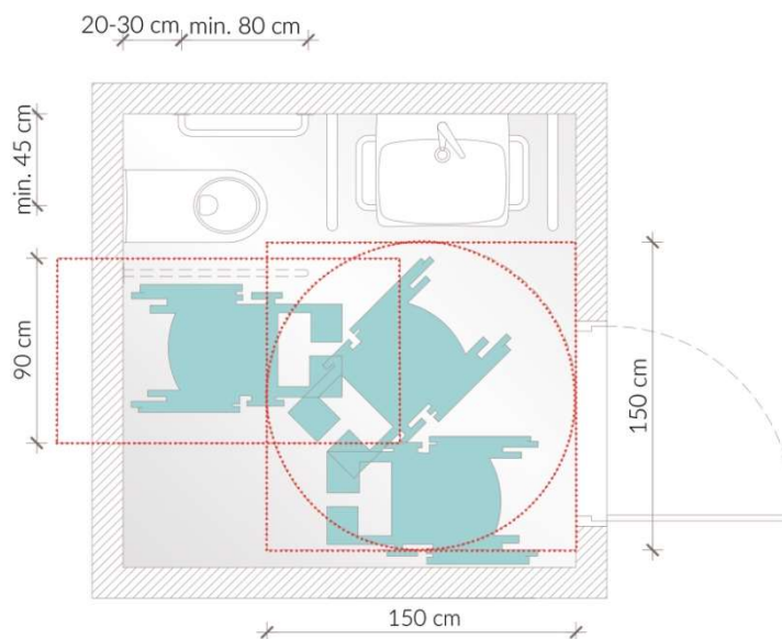
Rys. 53 Toaleta przeznaczona dla osób z niepełnosprawnościami
