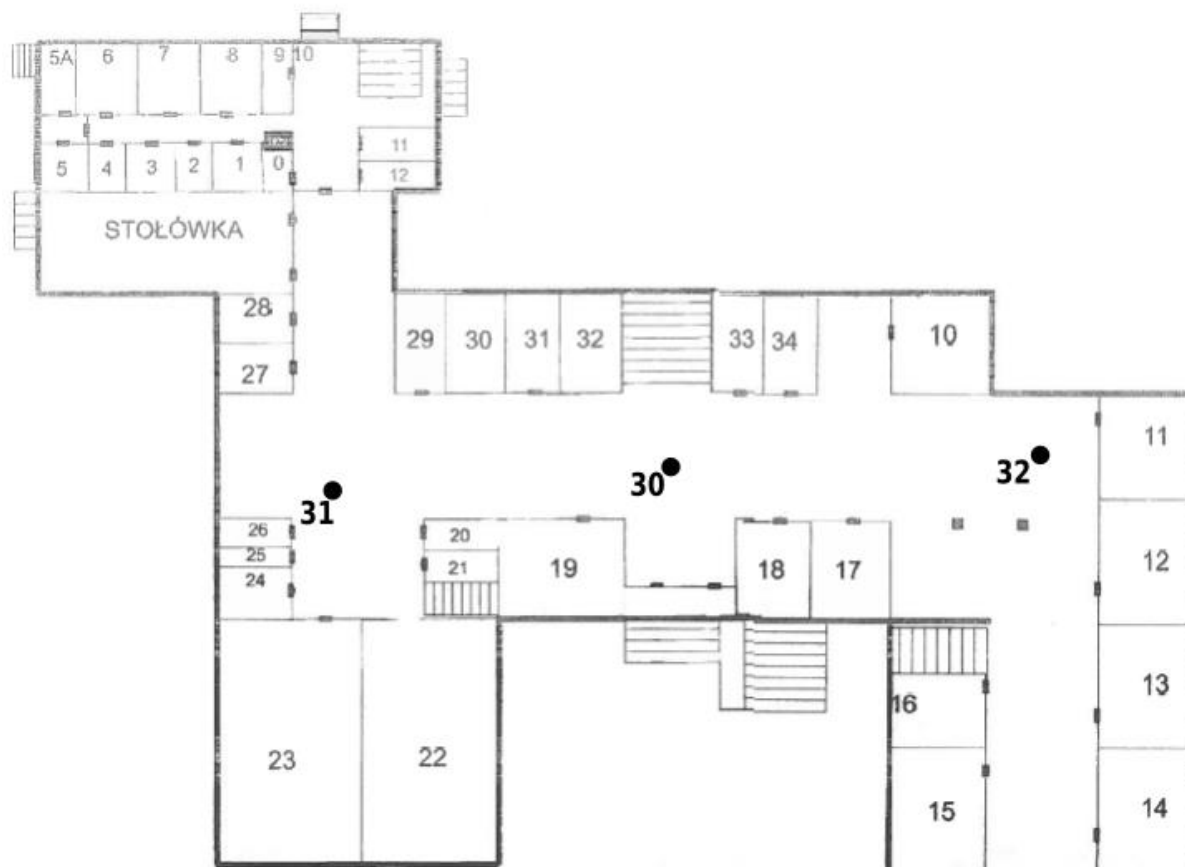
Rys. 1c: Plan rozmieszczenia punktów pomiarowych – piwnica
