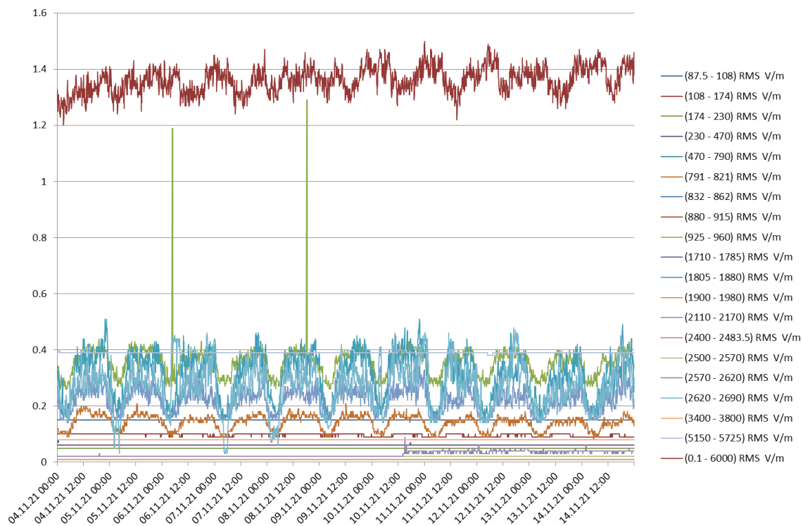
Rys. 5 Wyniki pomiarów dla 20 podzakresów częstotliwości – IŁ-PIB we Wrocławiu
