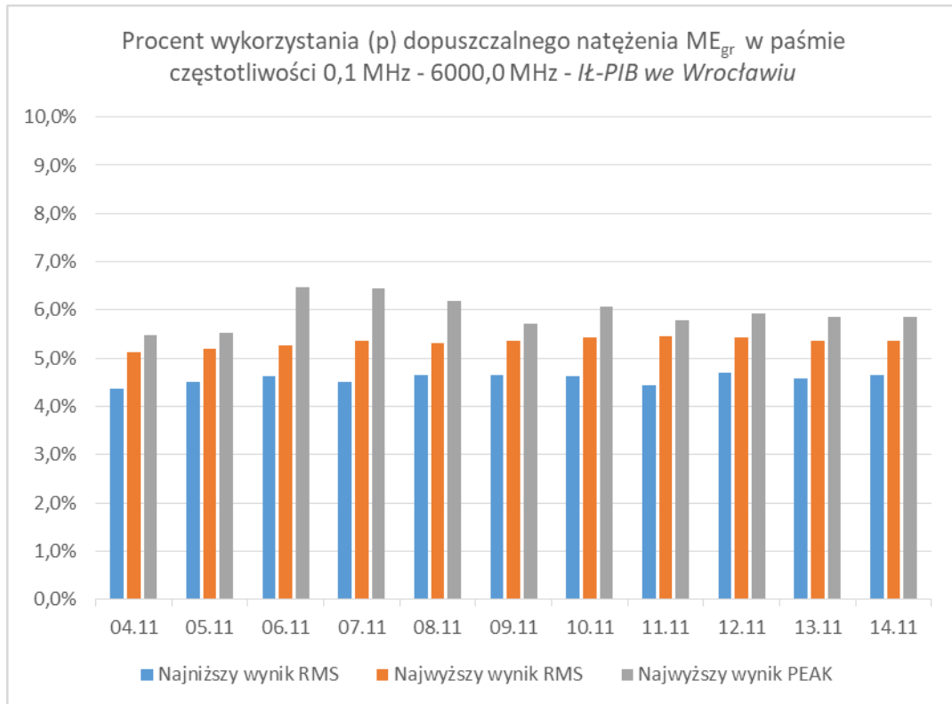
Rys. 26 Procentowe wykorzystanie dopuszczalnego natężenia w zakresie częstotliwości: 0,1 MHz – 6000,0 MHz – IŁ-PIB we Wrocławiu
