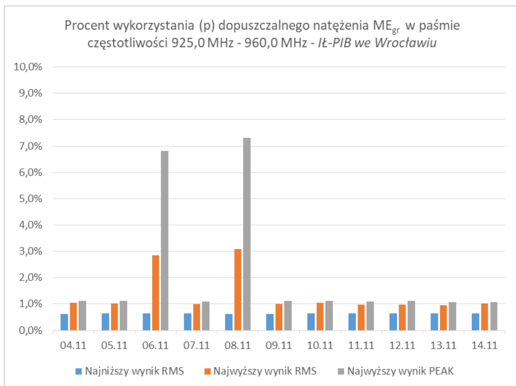
Rys. 27 Procentowe wykorzystanie dopuszczalnego natężenia w zakresie częstotliwości: 925,0 MHz – 960,0 MHz – IŁ-PIB we Wrocławiu
