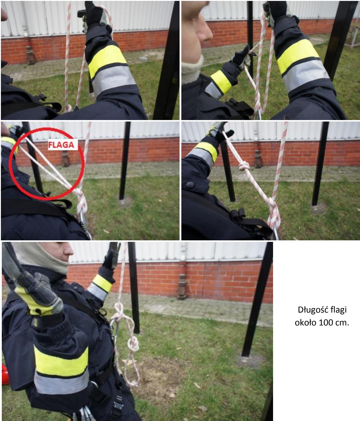
Rys. 24). Wiązanie węzła flagowego
