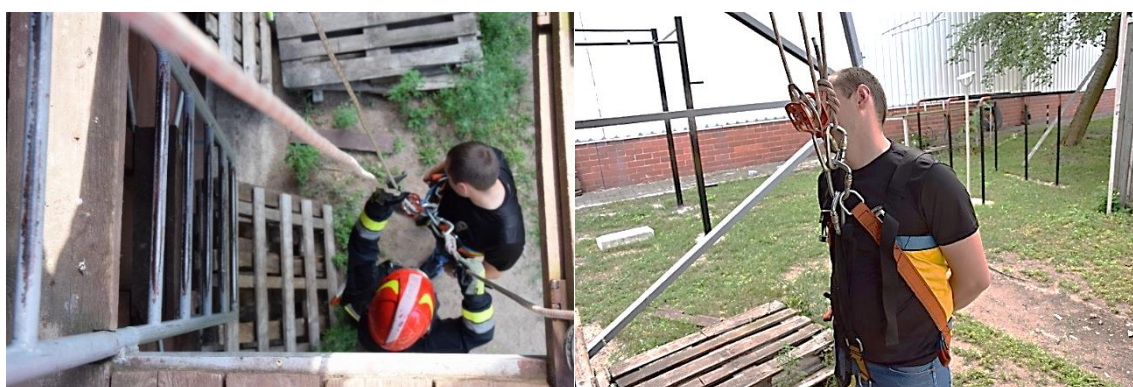
podjęcie poszkodowanego i przygotowanie do transportu w górę, technika dwóch lin
