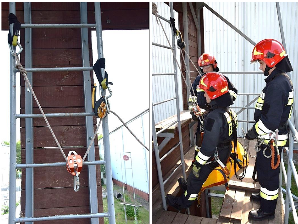
opuszczanie ratownika po poszkodowanego
