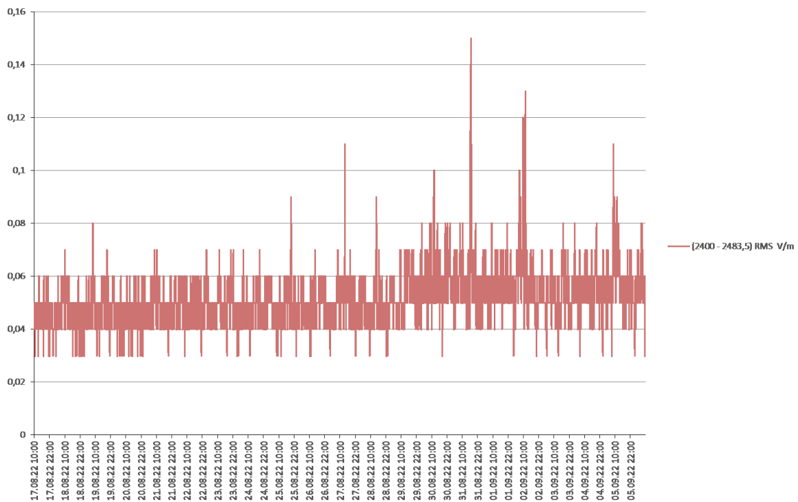
Rys. 19 Wyniki pomiarów w zakresie częstotliwości: 2400,0 MHz – 2483,5 MHz
