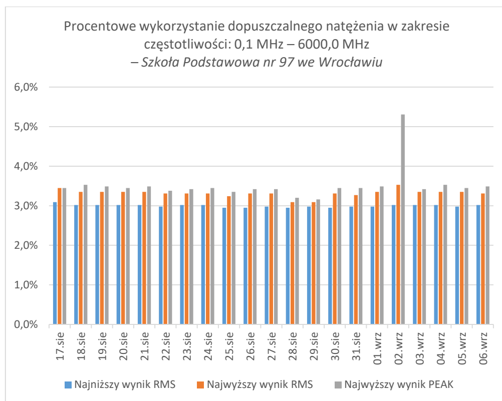
Rys. 25 Procentowe wykorzystanie dopuszczalnego natężenia w zakresie częstotliwości: 0,1 MHz – 6000,0 MHz – Szkoła Podstawowa nr 97 we Wrocławiu
