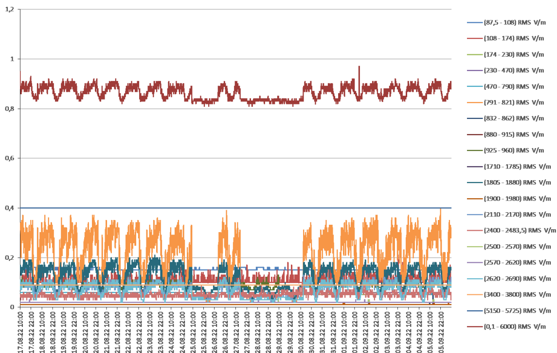
Rys. 4 Wyniki pomiarów dla 20 podzakresów częstotliwości – Szkoła Podstawowa nr 97 we Wrocławiu
