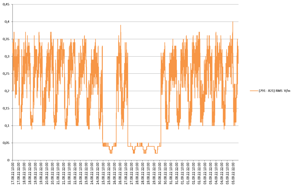
Rys. 11 Wyniki pomiarów w zakresie częstotliwości: 791,0 MHz – 821,0 MHz
