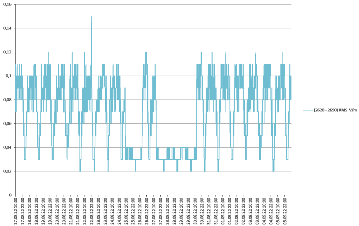
Rys. 22 Wyniki pomiarów w zakresie częstotliwości: 2620,0 MHz – 2690,0 MHz
