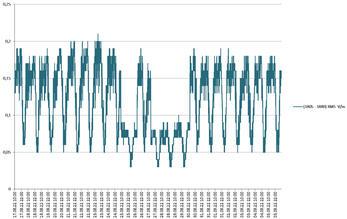
Rys. 16 Wyniki pomiarów w zakresie częstotliwości: 1805,0 MHz – 1880,0 MHz
