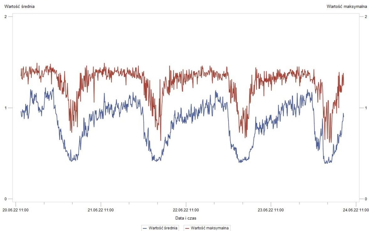
Rys. 5 Wyniki pomiarów – Szkoła Podstawowa nr 12 w Gdyni w dniach 20–24.06.2022 r.
