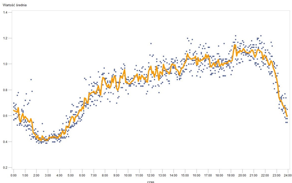
Rys. 6 Wyniki pomiarów – Szkoła Podstawowa nr 12 w Gdyni – średnia za okres 24 godzin
