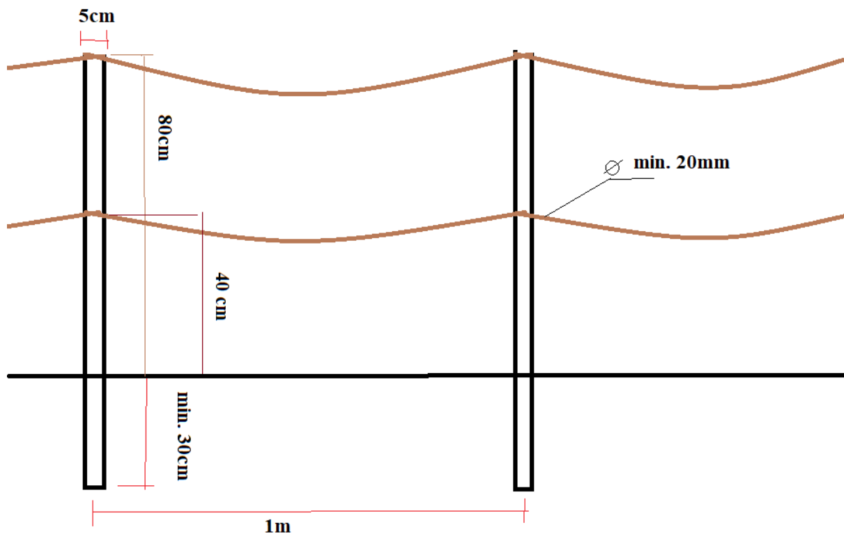
Ryc. 1. Schemat budowy barierki.
