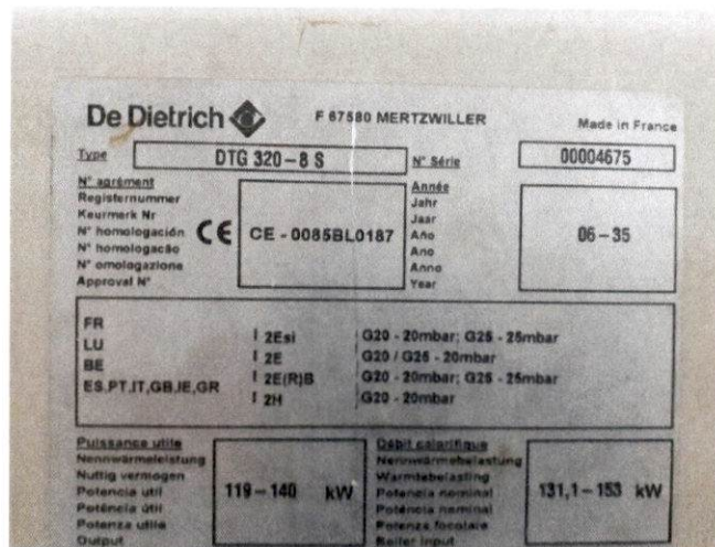
Rys. 2. Tabliczka znamionowa znajdująca się na obecnym kotle gazowym
