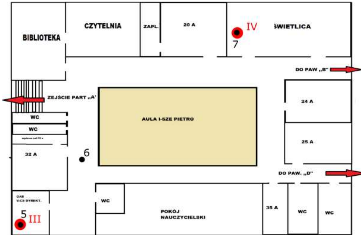
Rys. 1c: Plan rozmieszczenia punktów pomiarowych – pawilon A, I piętro, kolorem czerwonym oznaczono lokalizacje punktów dostępnych
