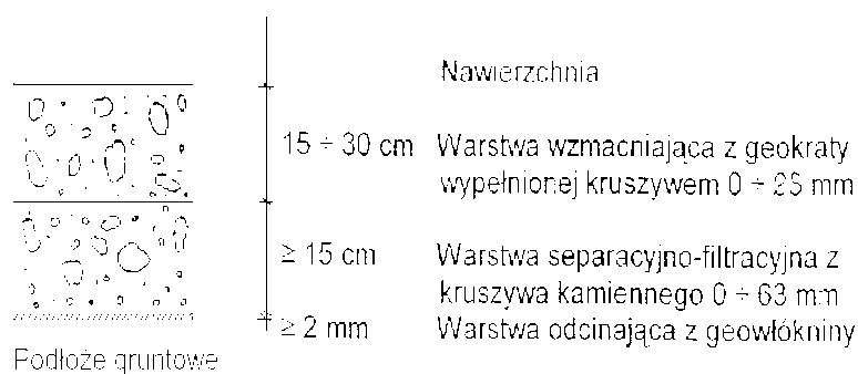
Rys. 3. Konstrukcja wzmocnienia podłoża pod nawierzchnią drogową za pomocą geokraty przestrzennej (przykład)
