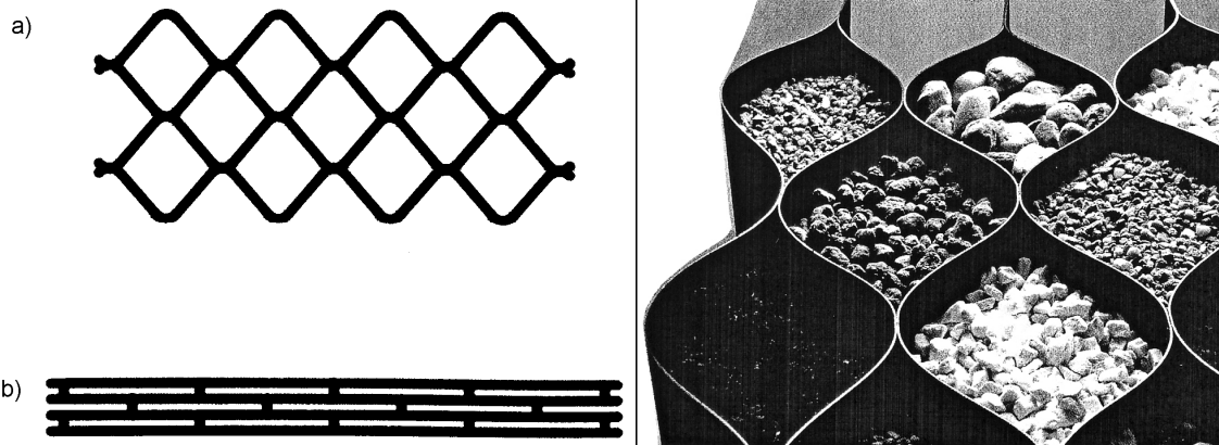
Rys. 1. Geokraty w pozycji rozłożonej i złożonej
