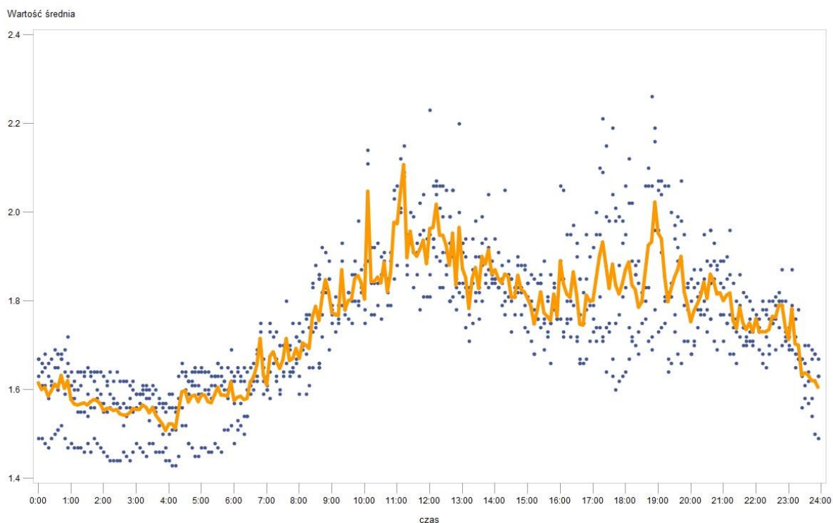
Rys. 6 Wyniki pomiarów – Zespół Szkół Mistrzostwa Sportowego w Gorzowie Wielkopolskim – średnia za okres 24 godzin
