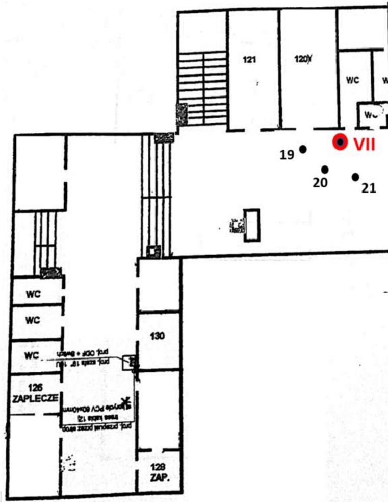
Rys. 1e: Plan rozmieszczenia punktów pomiarowych –I Piętro, kolorem czerwonym oznaczono lokalizację punktów dostępnych
