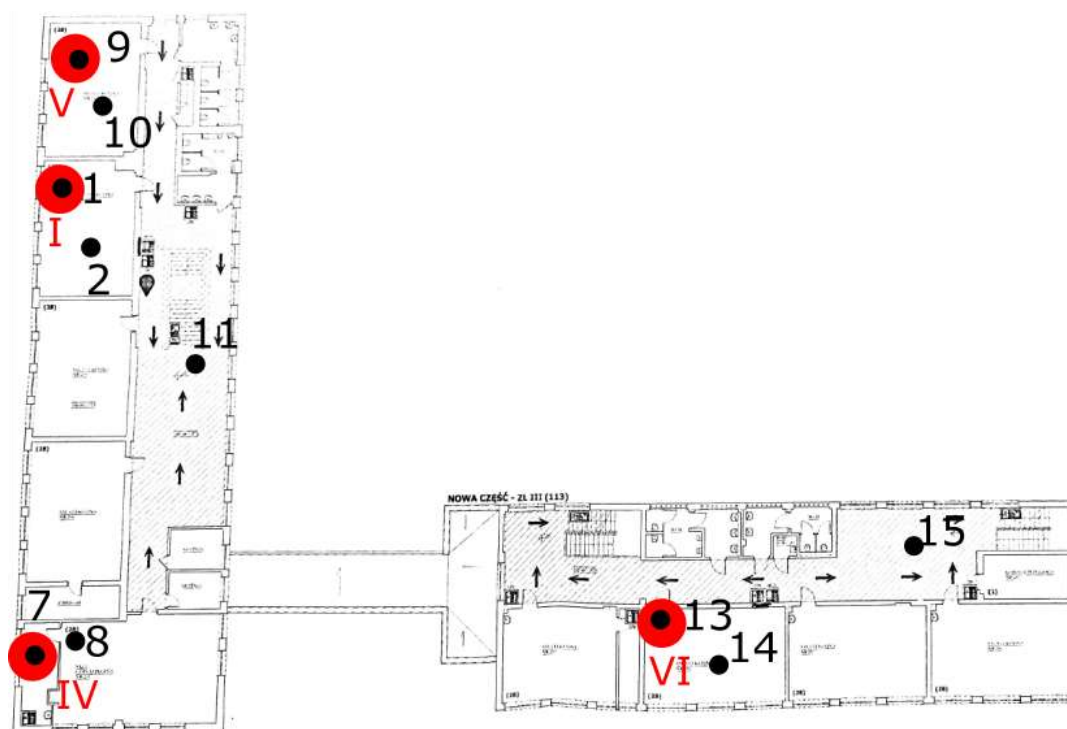
Rys. 1c: Plan rozmieszczenia punktów pomiarowych – II piętro, kolorem czerwonym oznaczono lokalizacje punktów dostępowych
