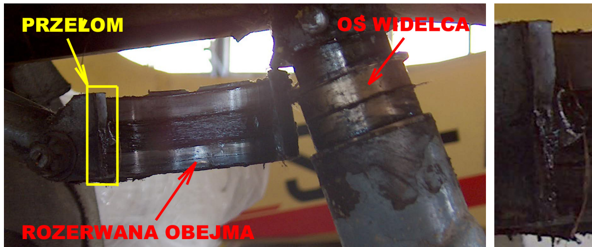
Fot.6a i 6b – Widok uszkodzeń z lewej strony kadłuba, po prawej (Fot.6b) zbliżenie przełomu obejmy.
