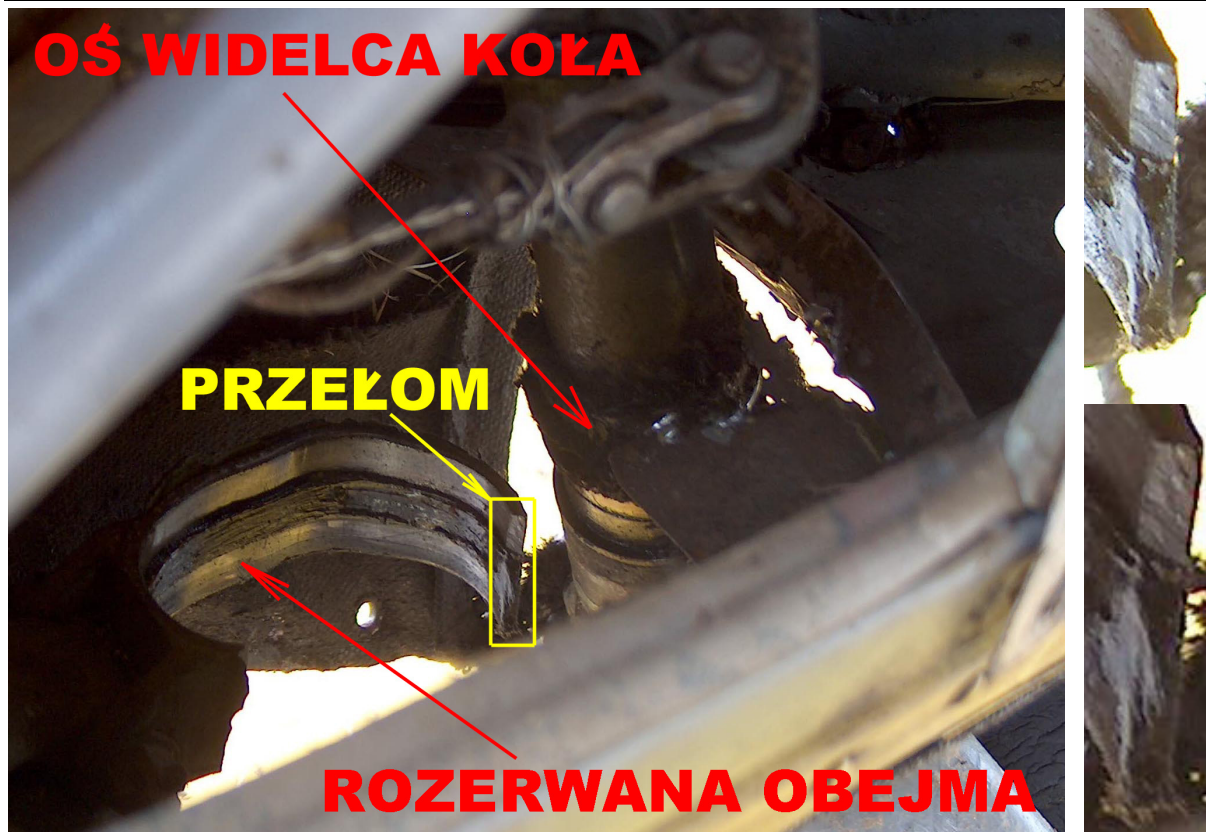
Fot.5a, 5b i 5c – Widok uszkodzeń z góry, po prawej dwa zbliżenia przełomu obejmy (Fot.5b i 5c).
