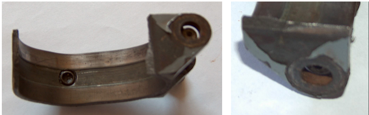
Fot.7a i 7b – Uszkodzona obejma po demontażu i oczyszczeniu.
